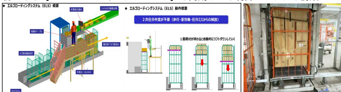
エルゴローディングシステム全体図と出荷カゴ台車への自動積み付け
